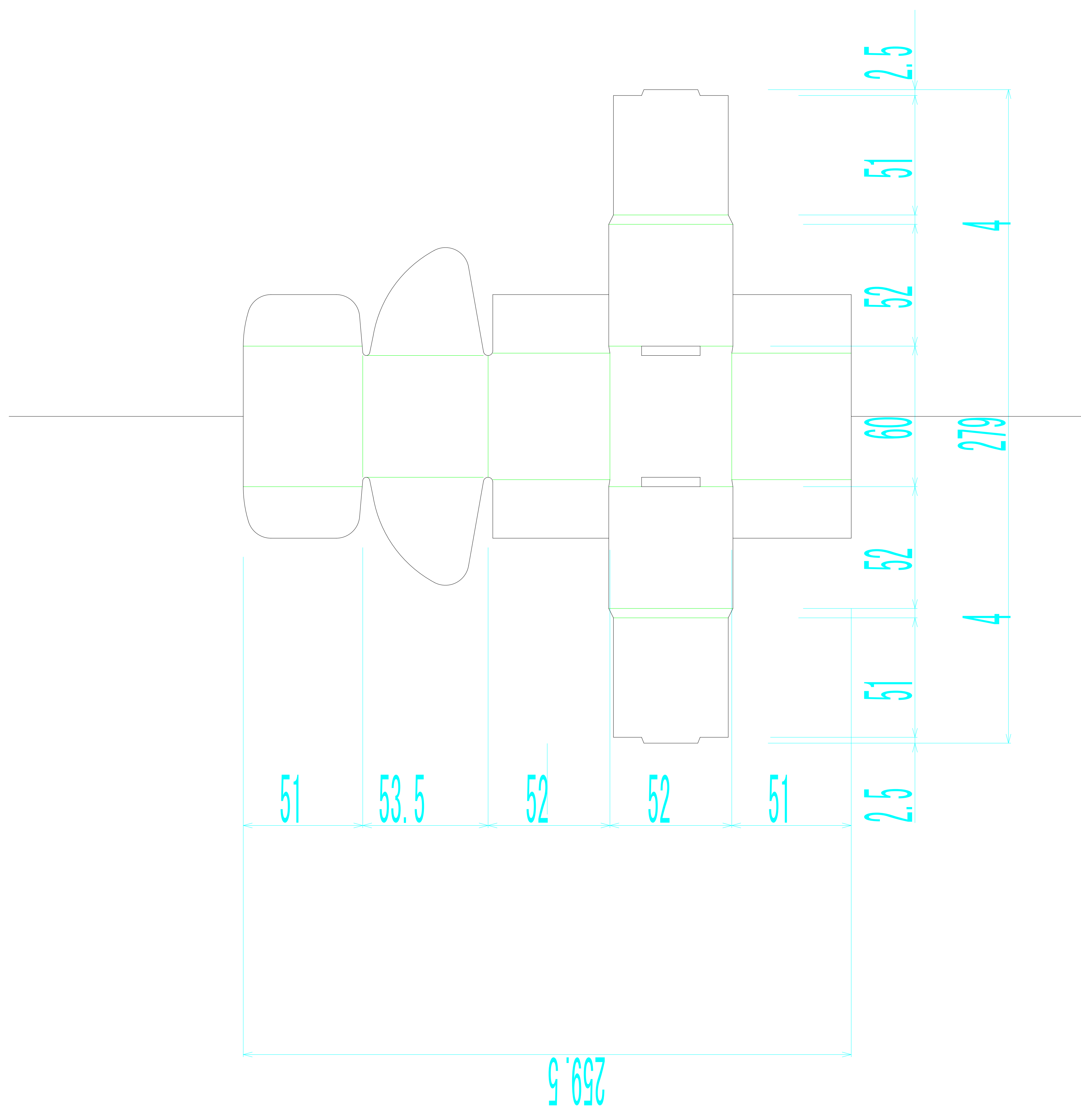
G4002 N式(額縁) EF/1.5mm
